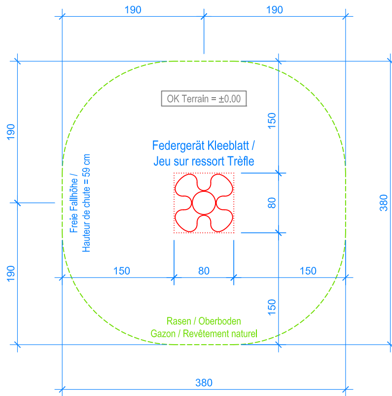
GRUNDRISS / PLAN 1:50
