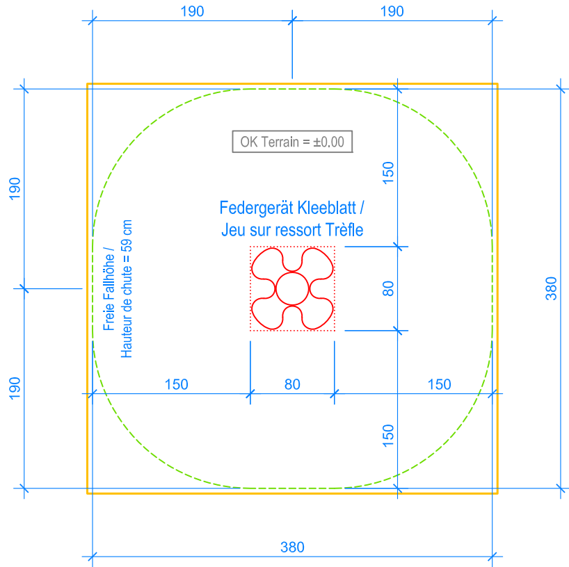
GRUNDRISS / PLAN 1:50
