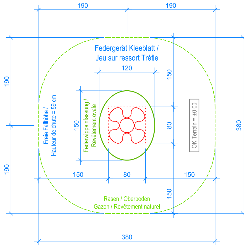
GRUNDRISS / PLAN 1:50
