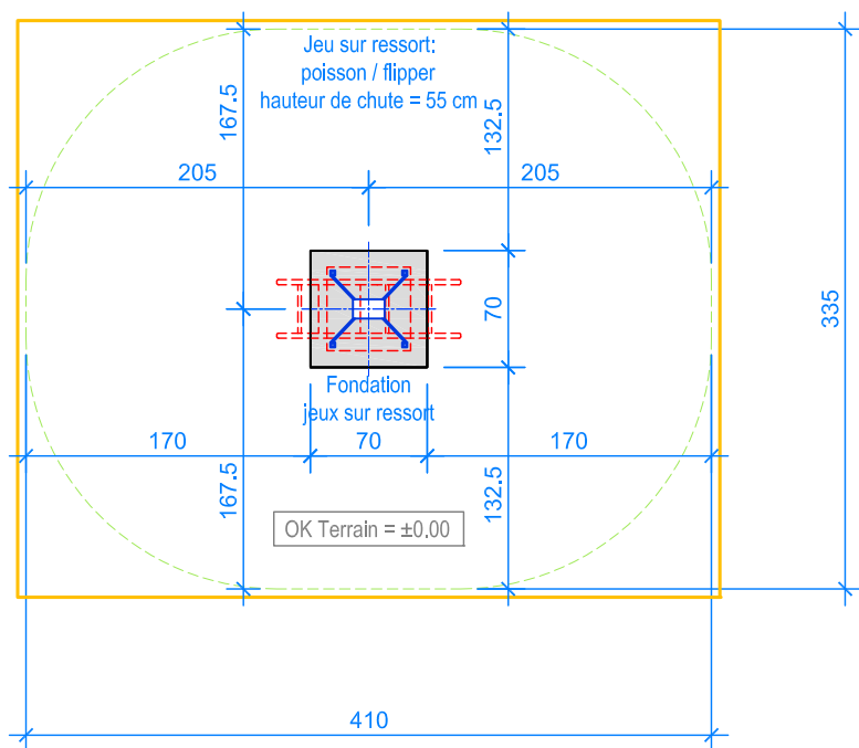
PLAN 1:50
