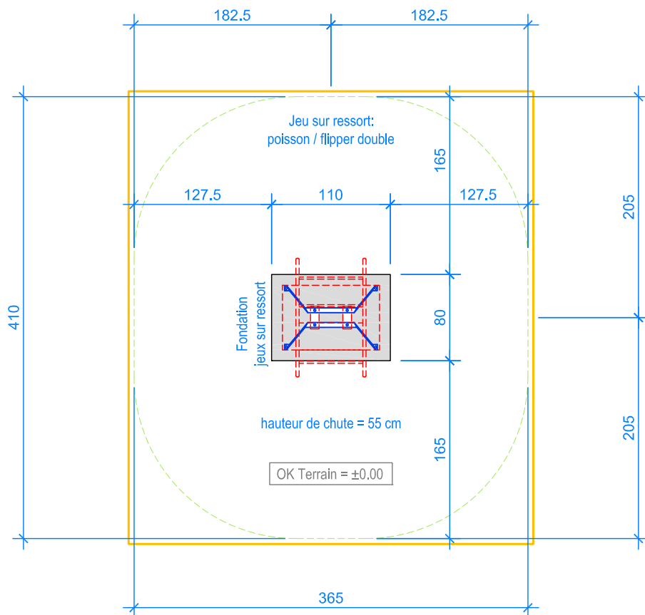
PLAN 1:50
