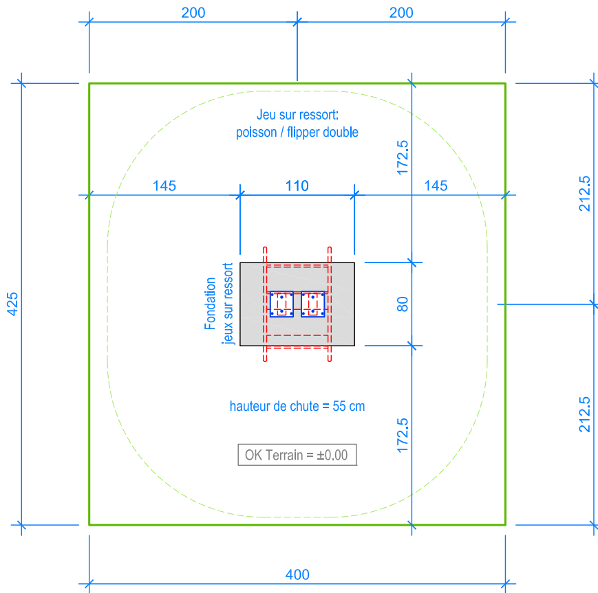
PLAN 1:50
