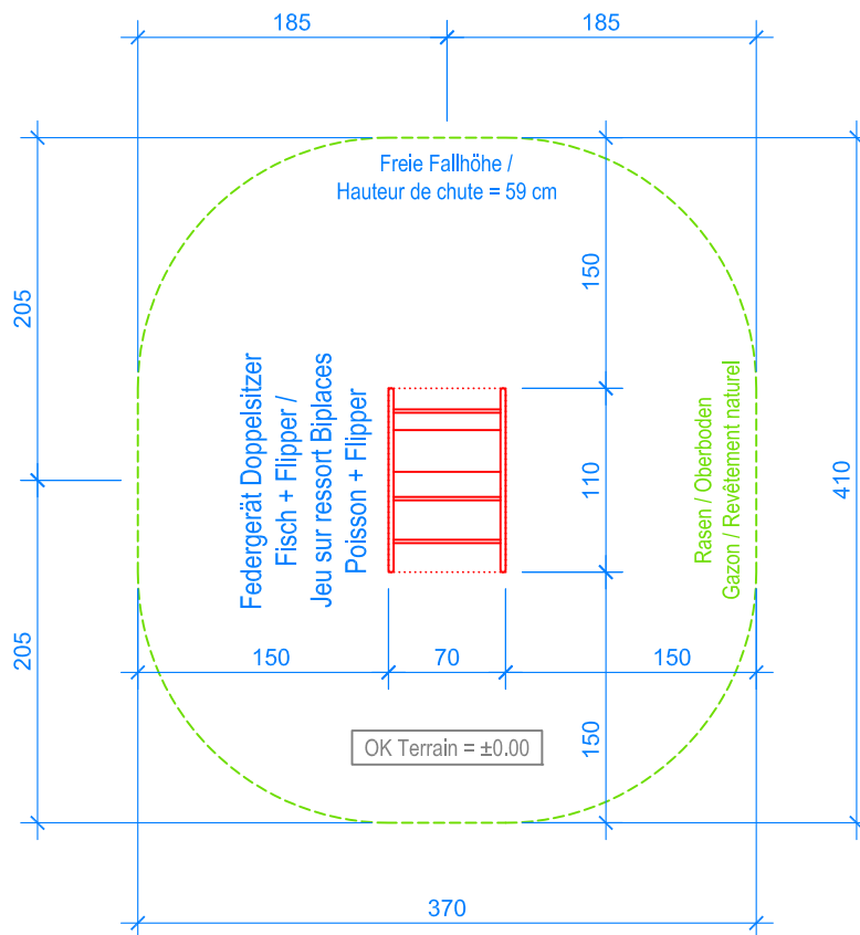
GRUNDRISS / PLAN 1:50
