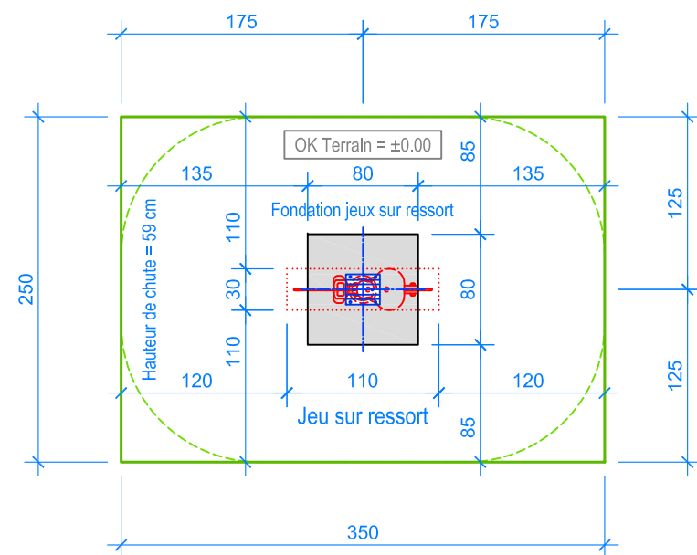
PLAN 1:50
