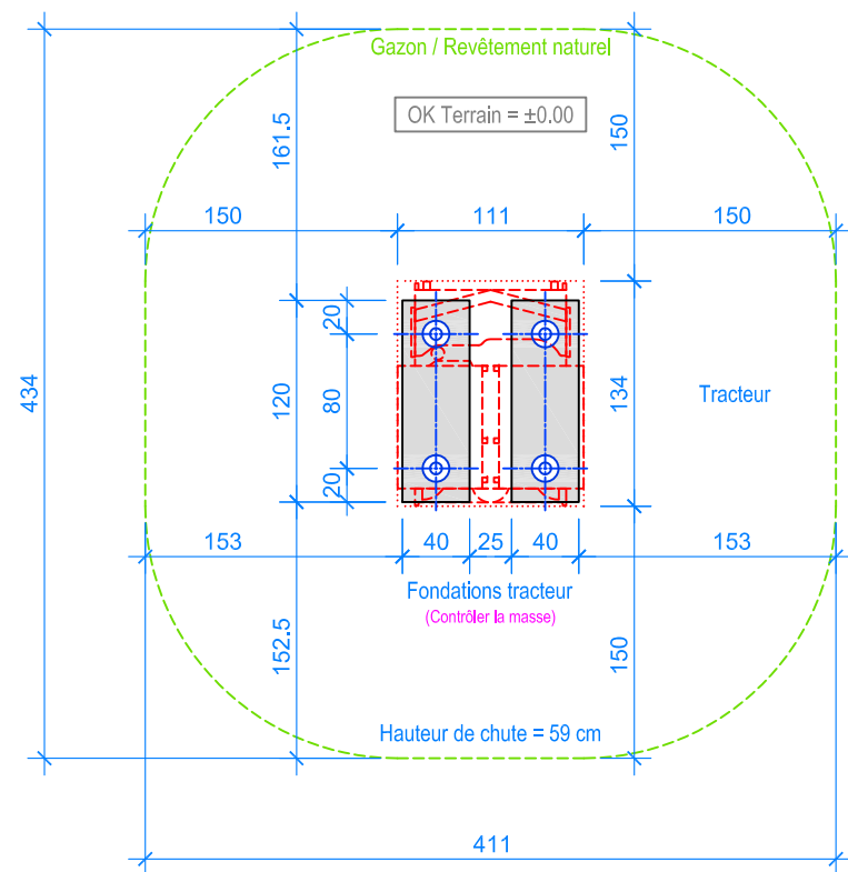
PLAN 1:50
