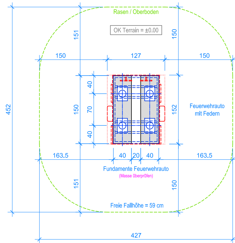
GRUNDRISS 1:50
