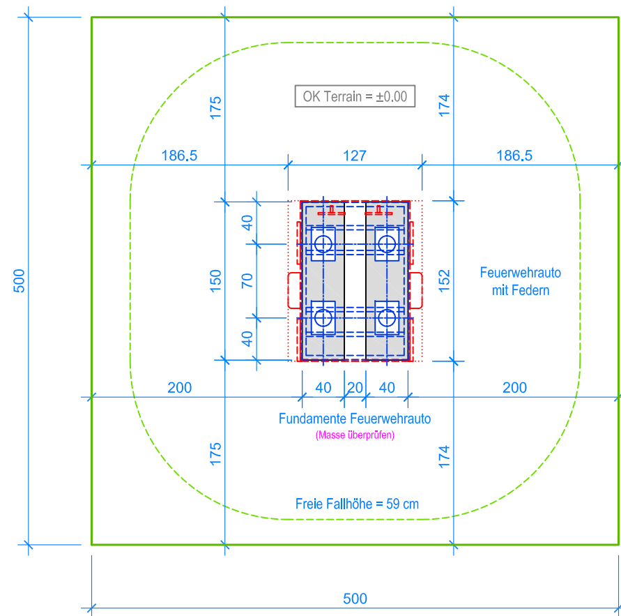
GRUNDRISS 1:50
