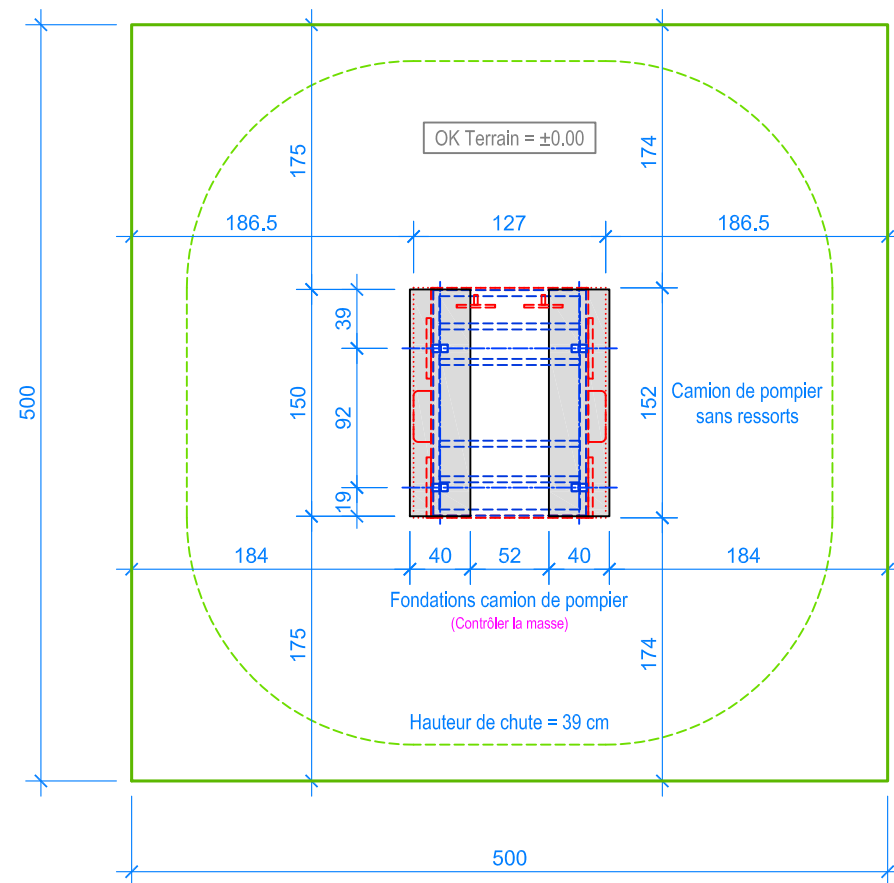
PLAN 1:50
