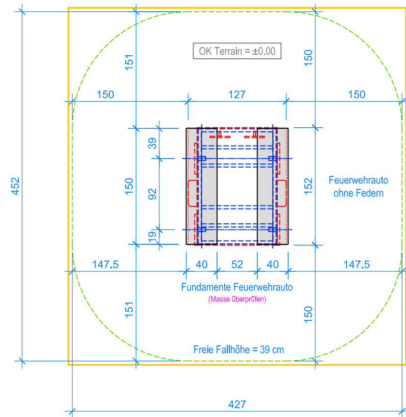
GRUNDRISS 1:50
