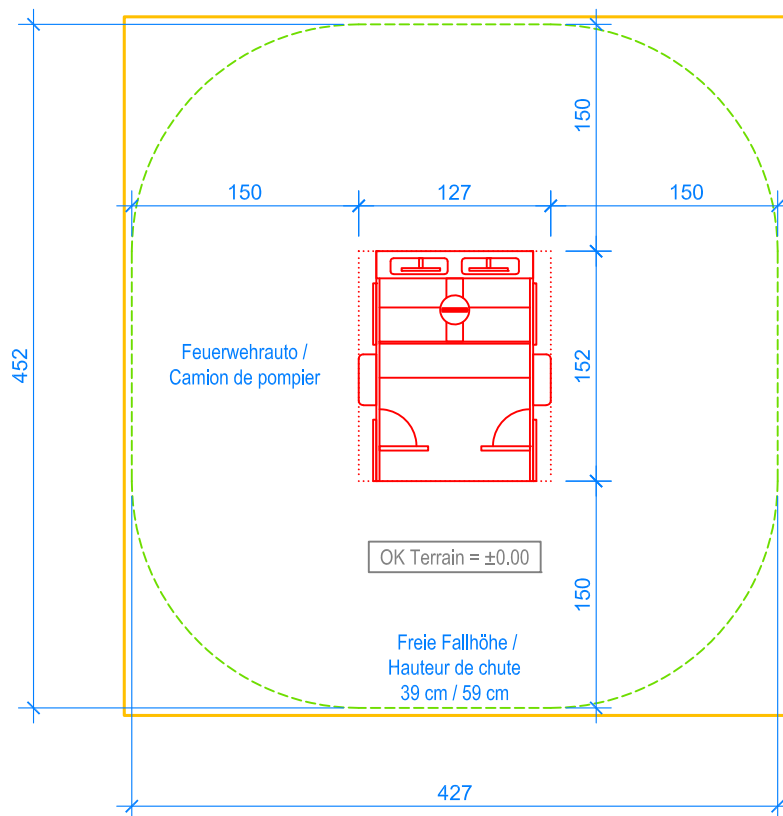
GRUNDRISS / PLAN 1:50
