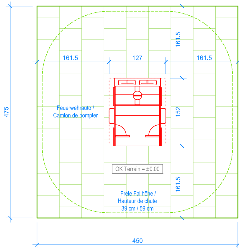
GRUNDRISS / PLAN 1:50
