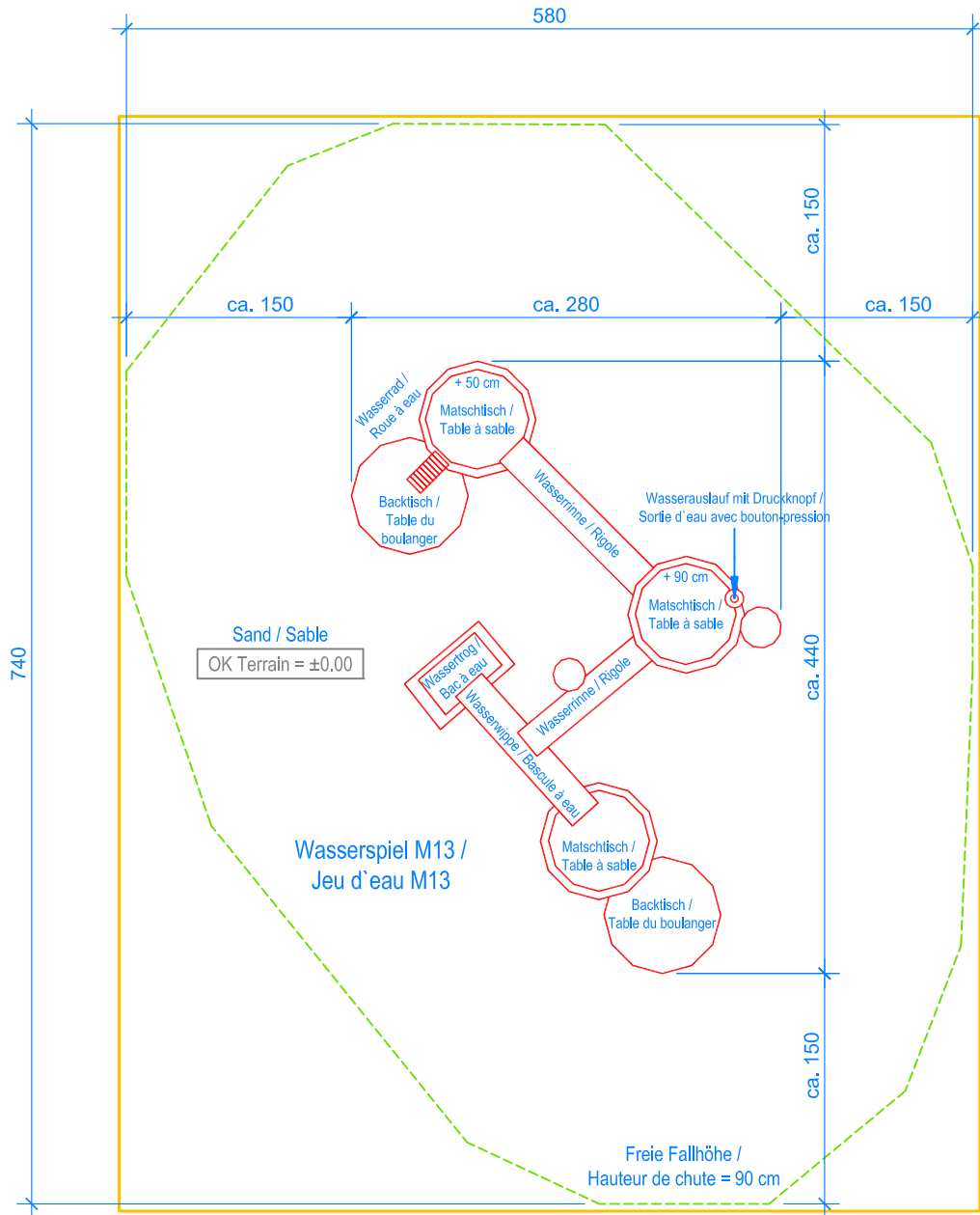
GRUNDRISS / PLAN 1:50
