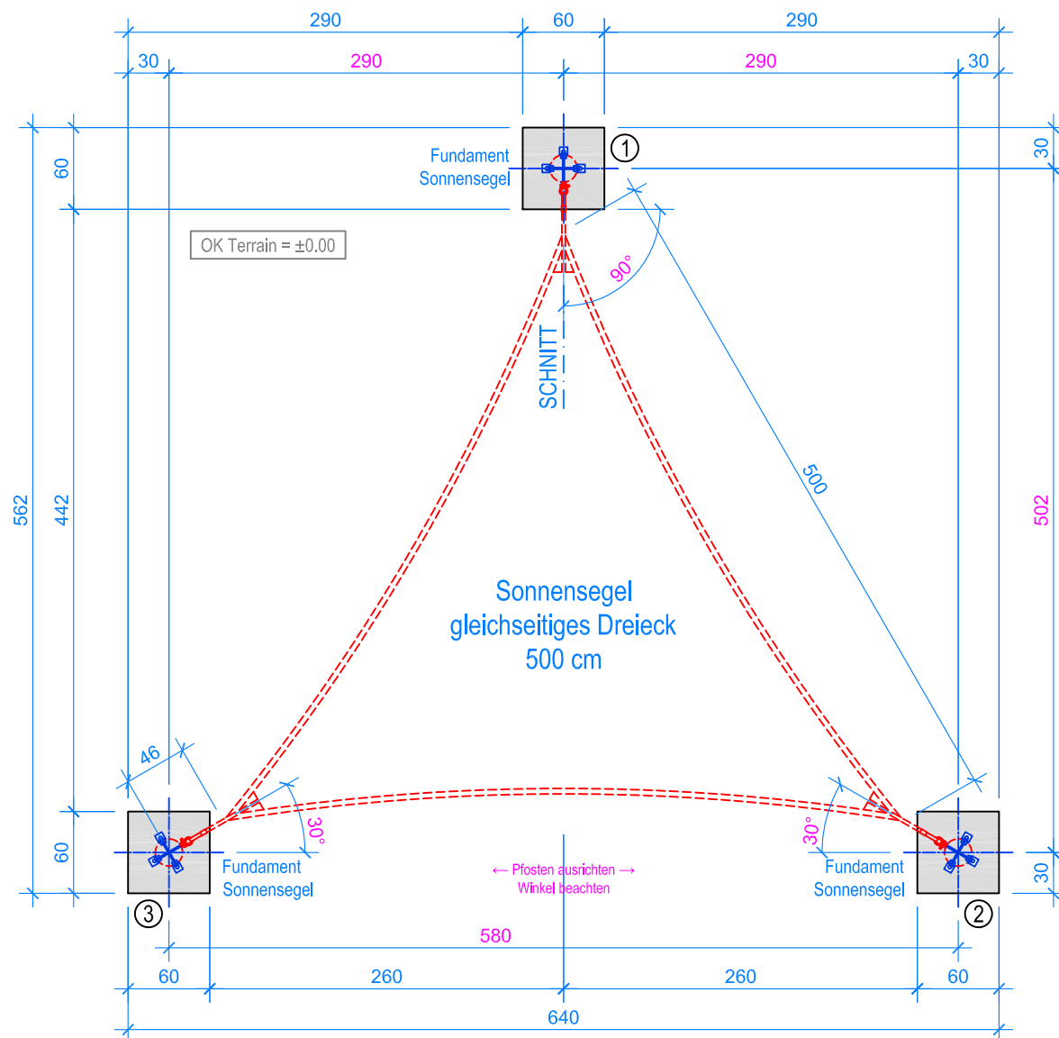
GRUNDRISS 1:50
