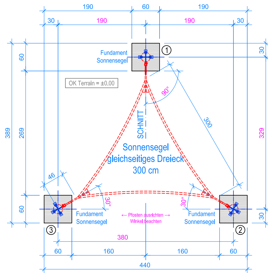
GRUNDRISS 1:50
