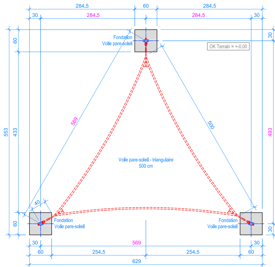
PLAN 1:50
