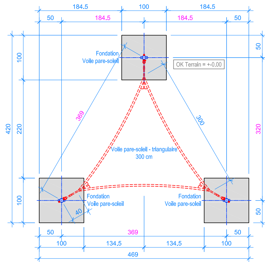
PLAN 1:50
