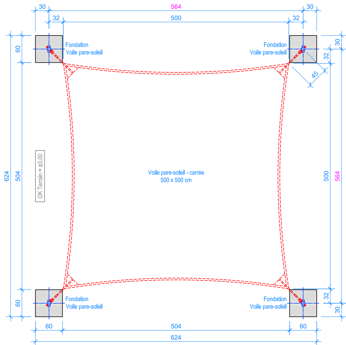
PLAN 1:50
