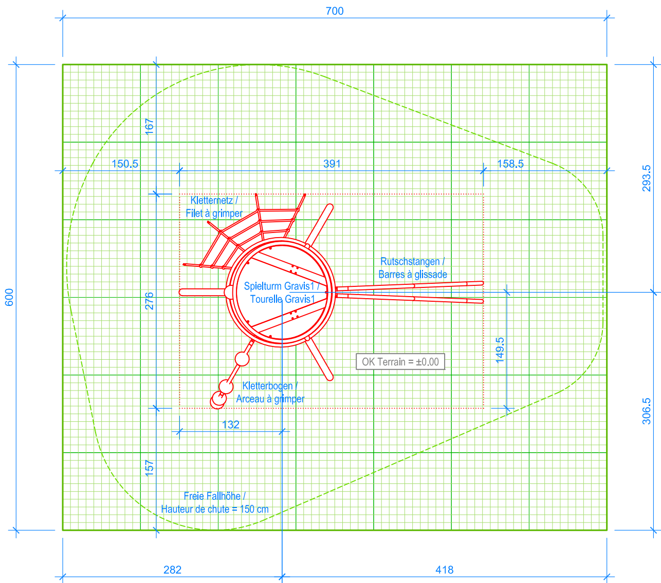
GRUNDRISS / PLAN 1:50
