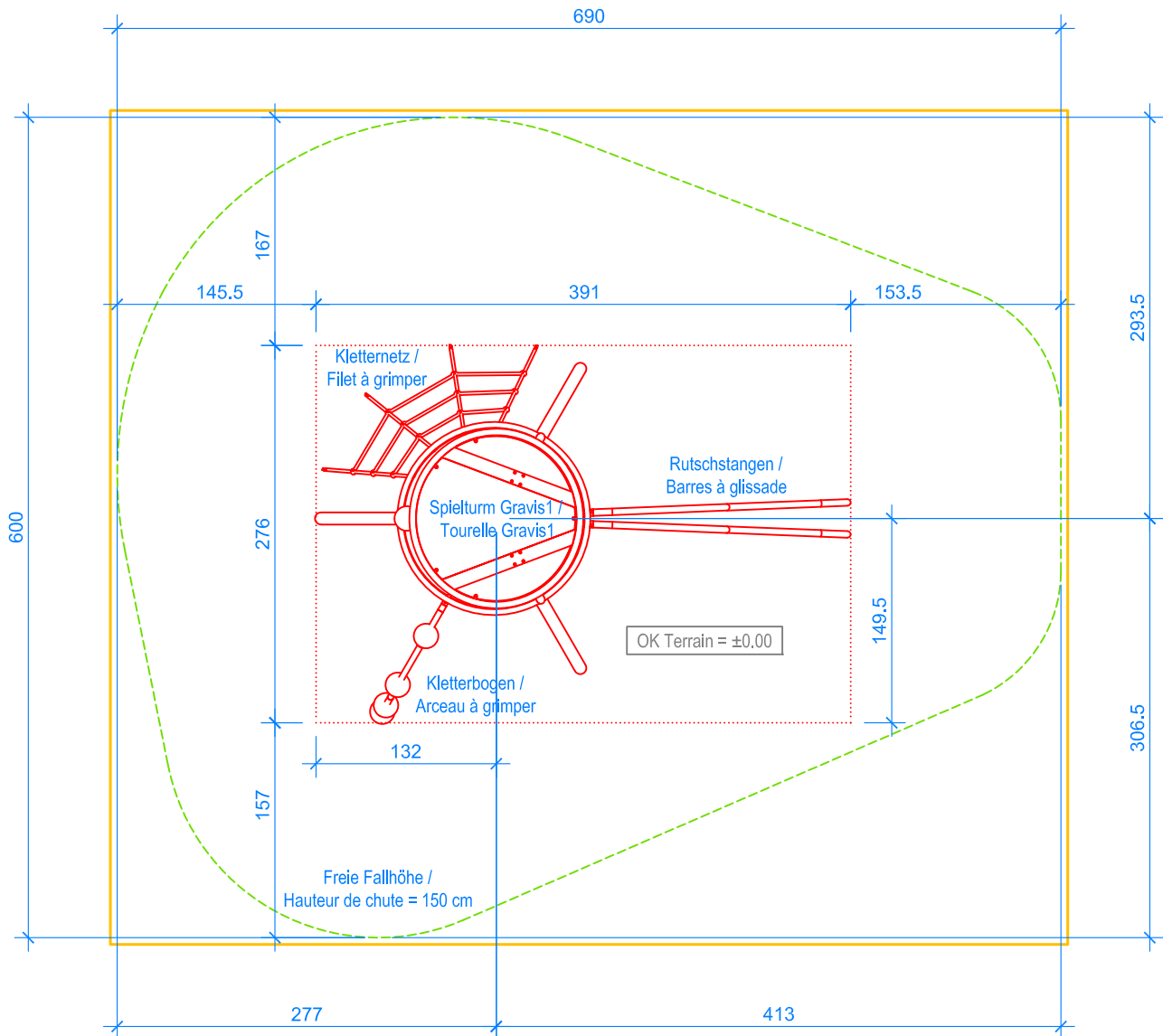
GRUNDRISS / PLAN 1:50
