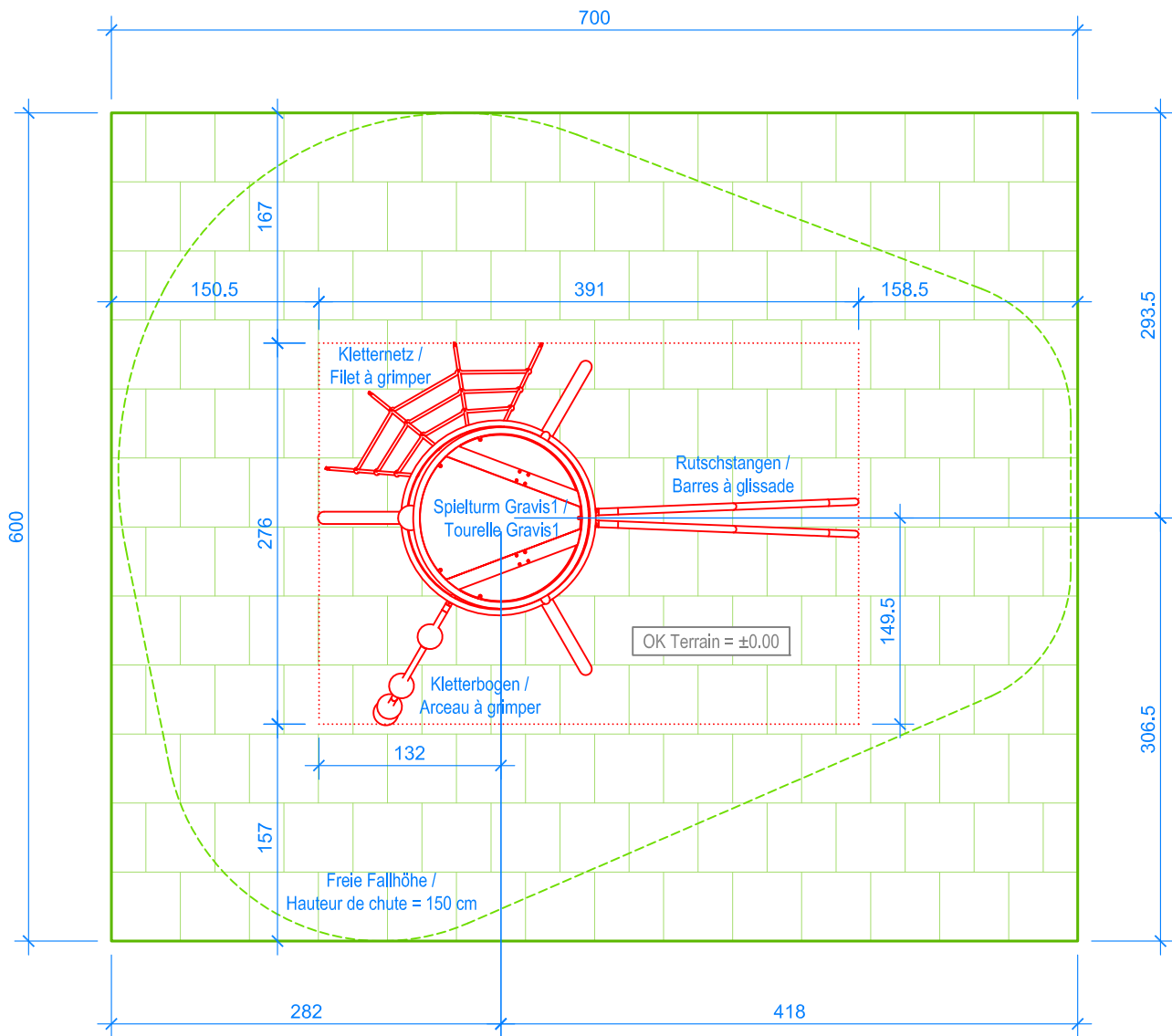
GRUNDRISS / PLAN 1:50
