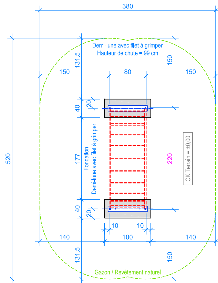
PLAN 1:50
