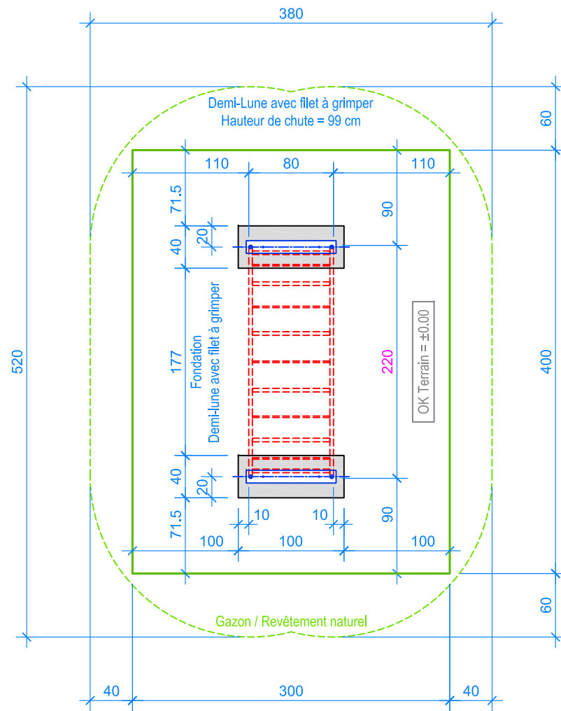
PLAN 1:50
