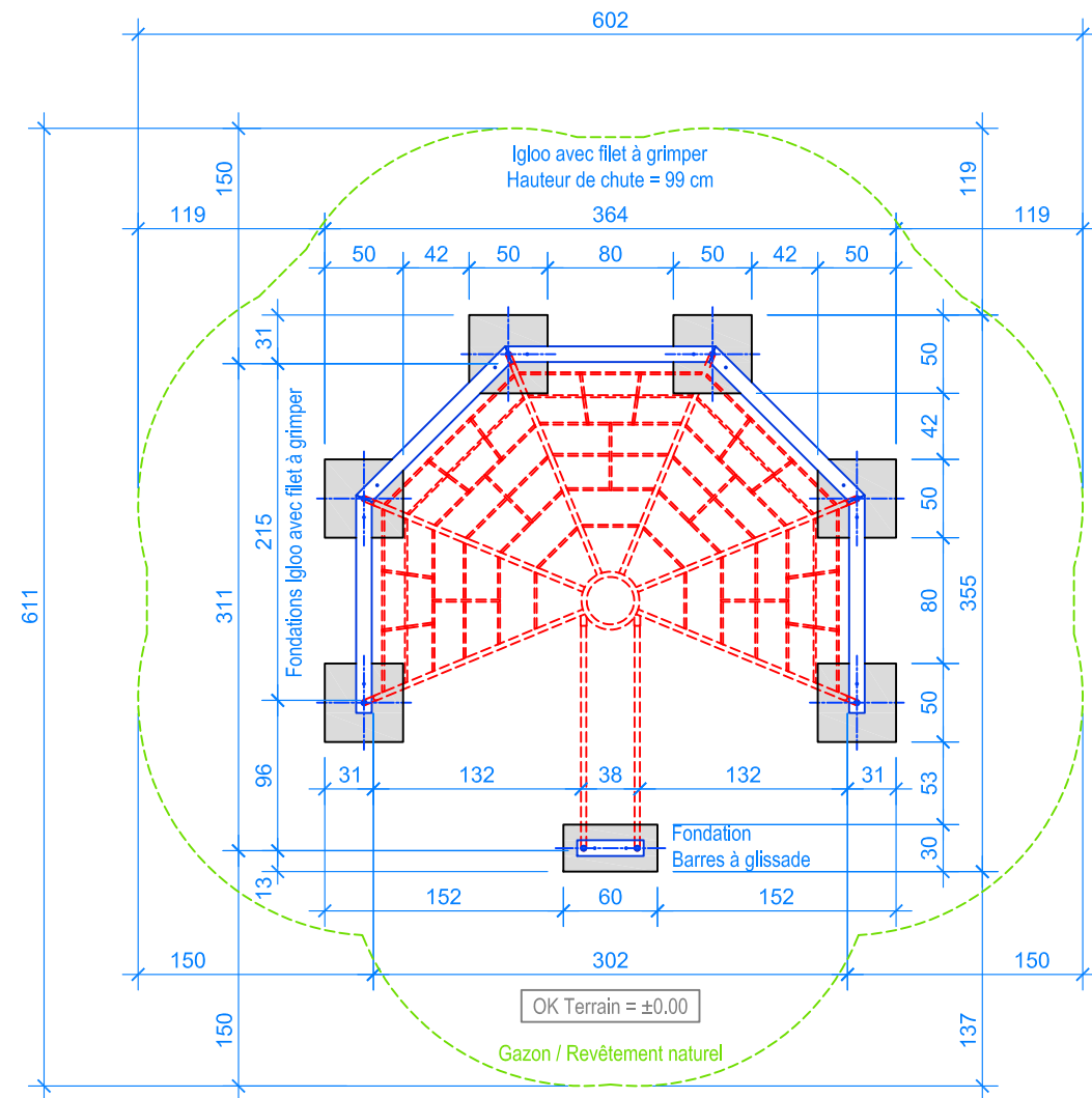
PLAN 1:50
