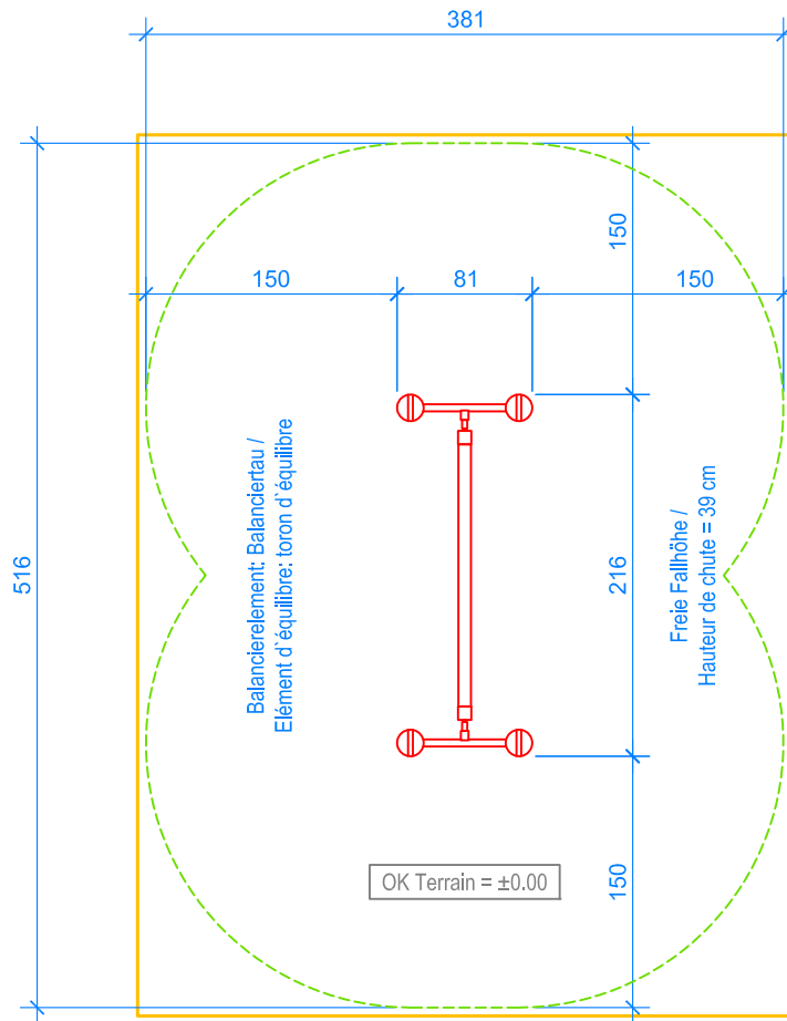
GRUNDRISS / PLAN 1:50
