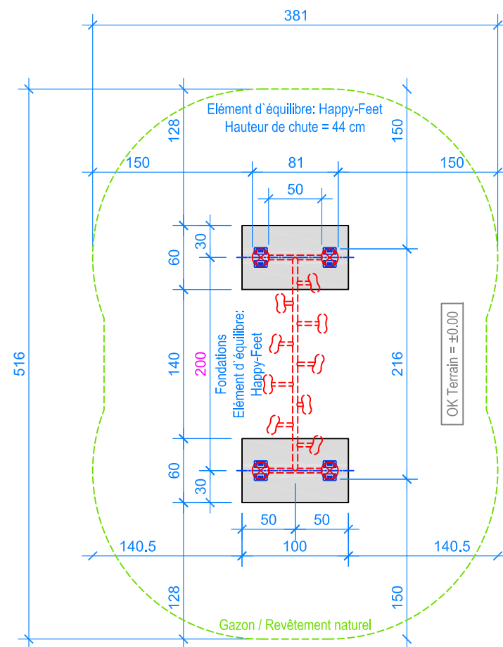
PLAN 1:50
