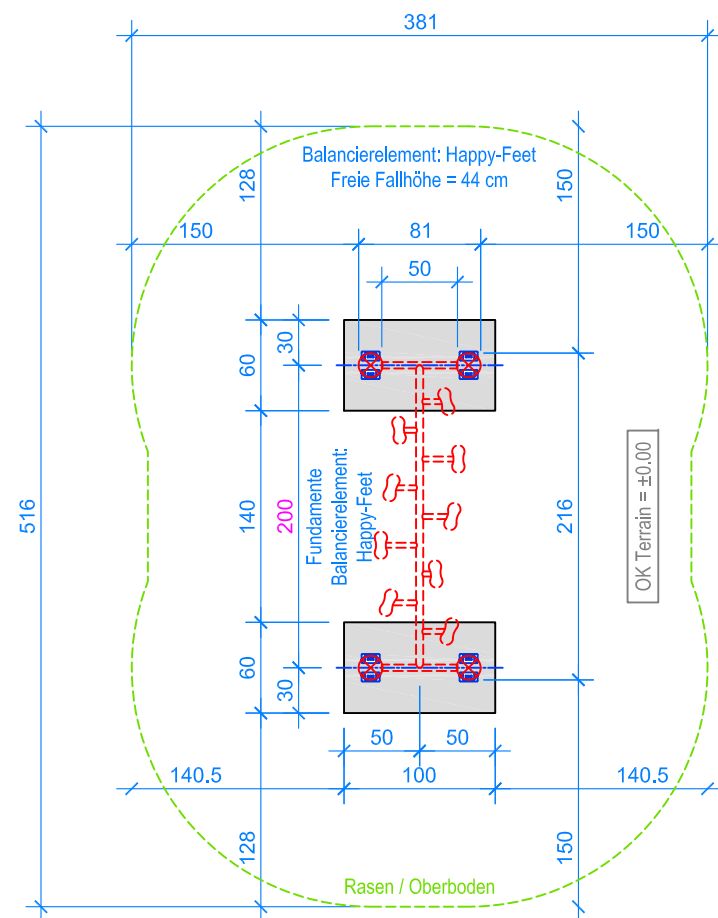
GRUNDRISS 1:50
