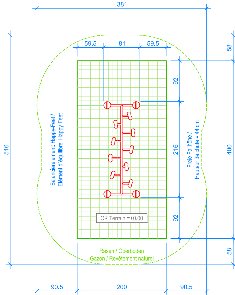
GRUNDRISS / PLAN 1:50
