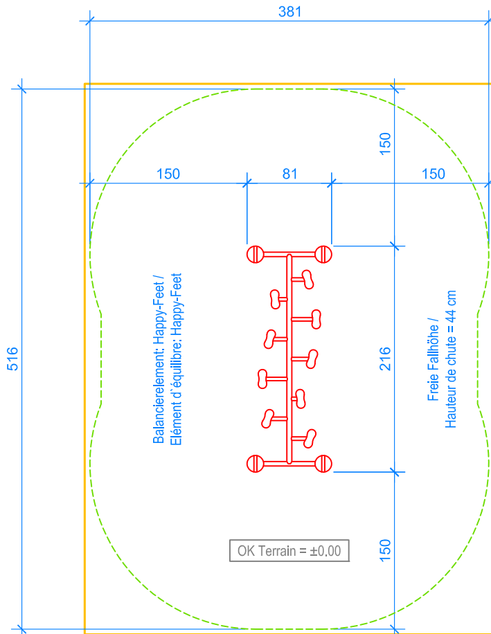
GRUNDRISS / PLAN 1:50
