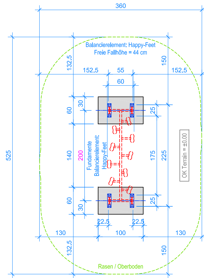
GRUNDRISS 1:50
