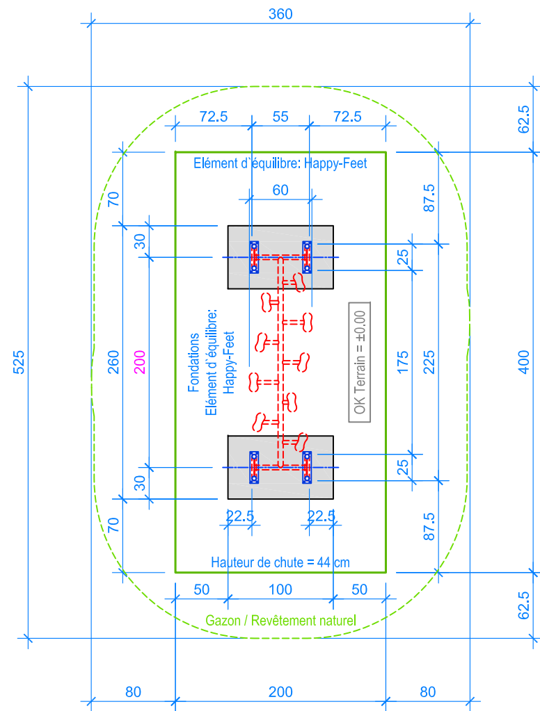
PLAN 1:50
