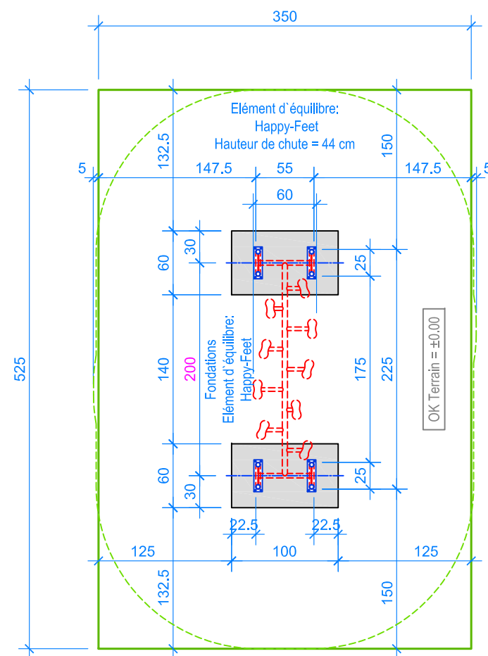
PLAN 1:50
