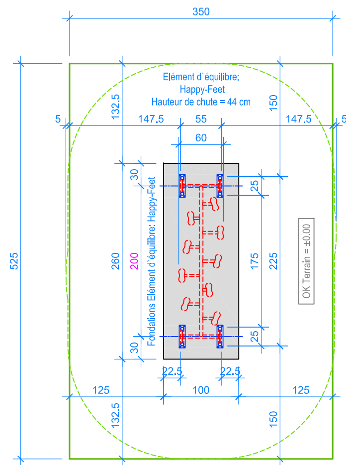
PLAN 1:50
