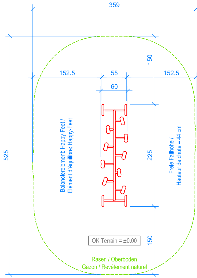
GRUNDRISS / PLAN 1:50
