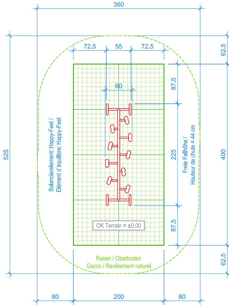
GRUNDRISS / PLAN 1:50
