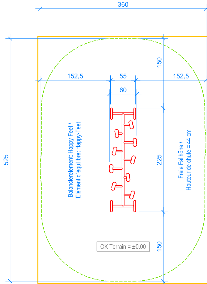
GRUNDRISS / PLAN 1:50
