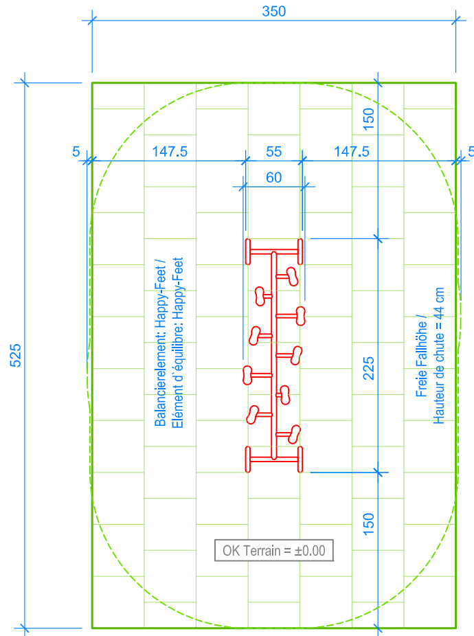
GRUNDRISS / PLAN 1:50
