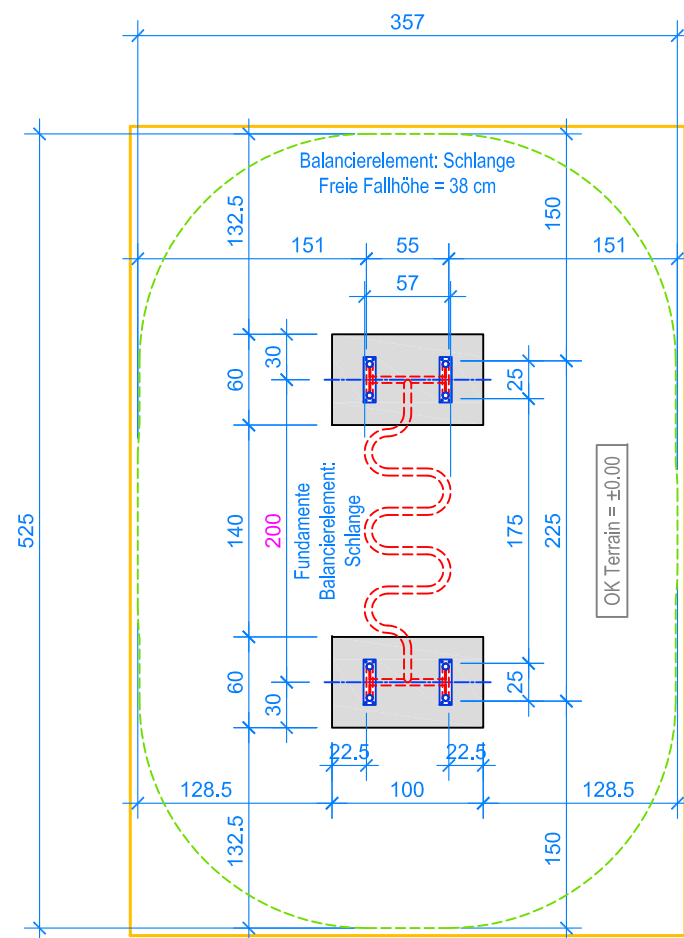
GRUNDRISS 1:50
