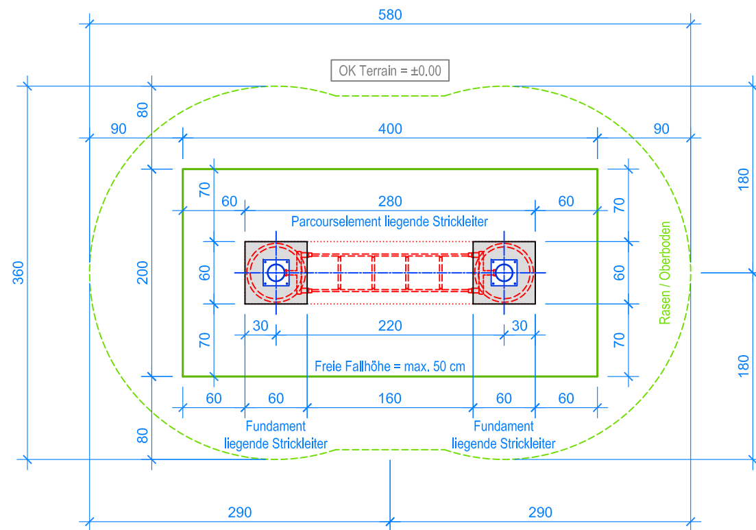
GRUNDRISS 1:50
