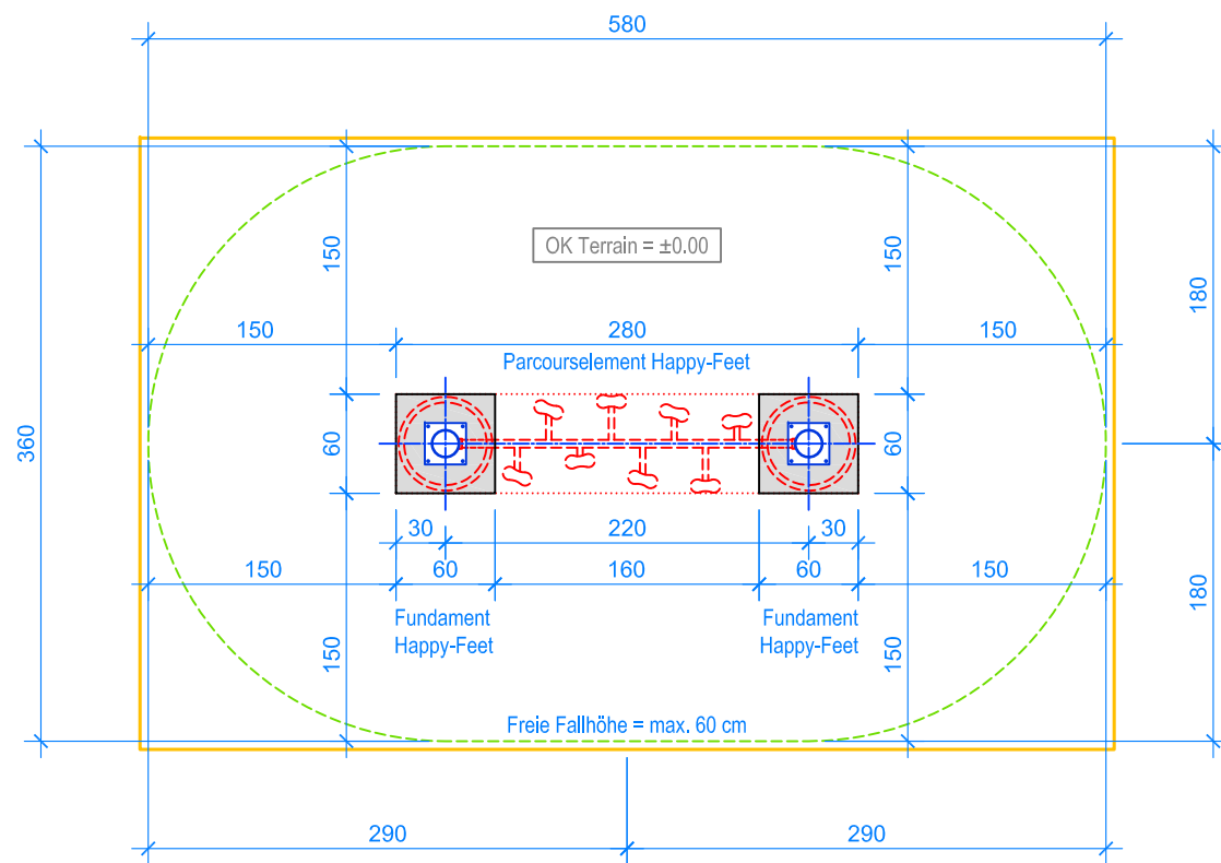
GRUNDRISS 1:50
