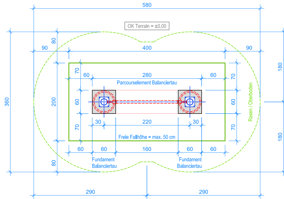
GRUNDRISS 1:50
