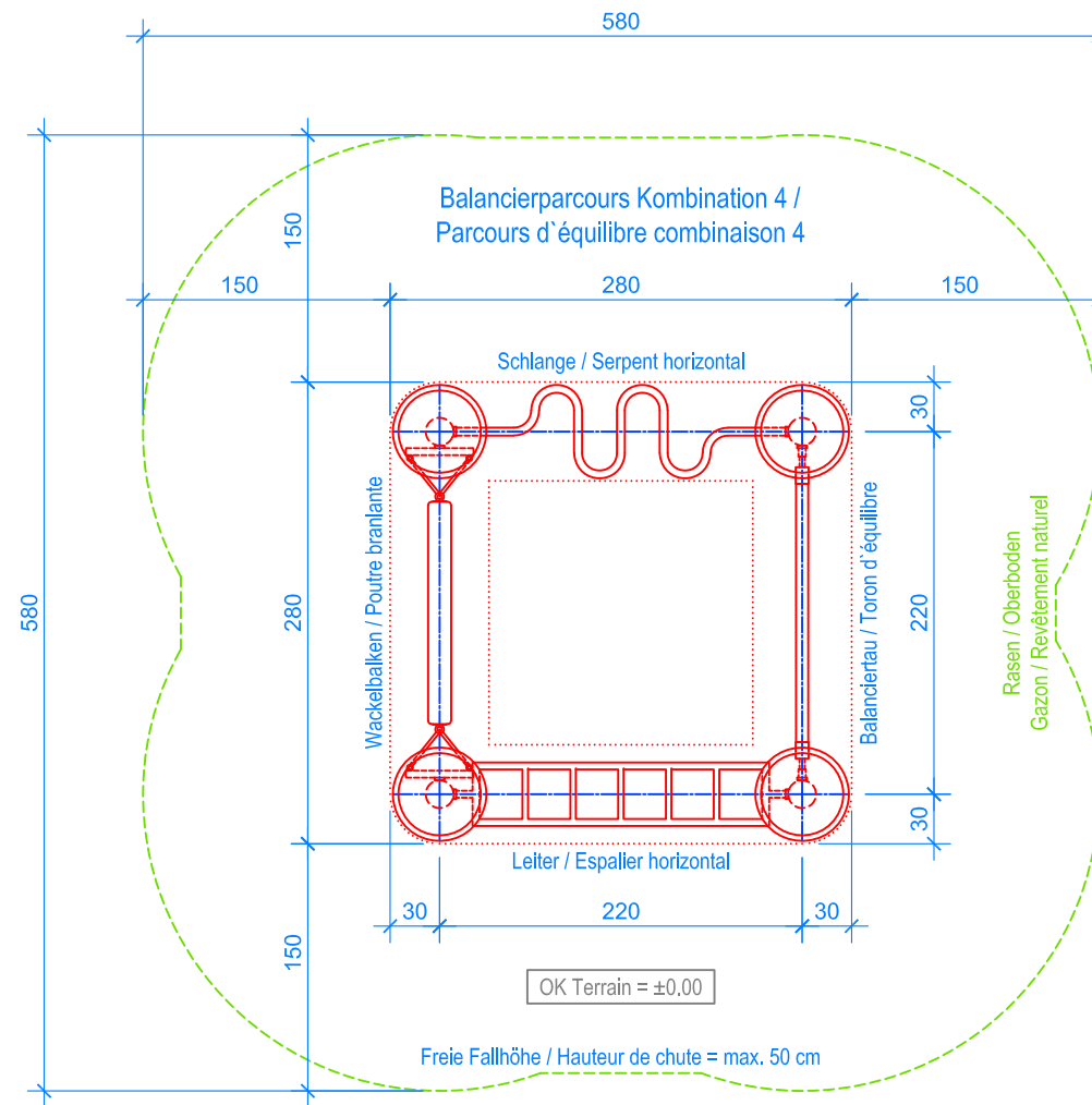
GRUNDRISS / PLAN 1:50
