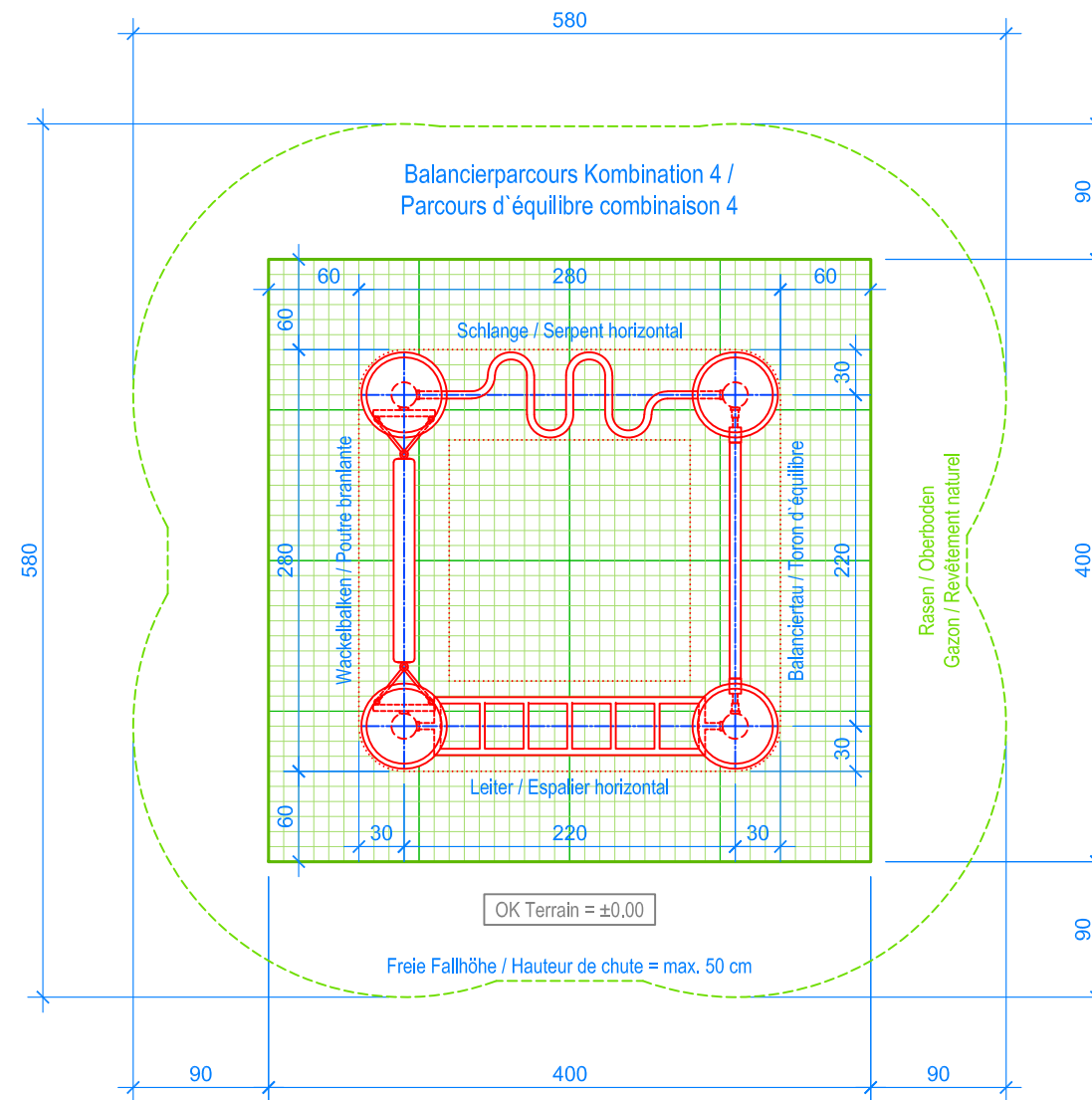
GRUNDRISS / PLAN 1:50
