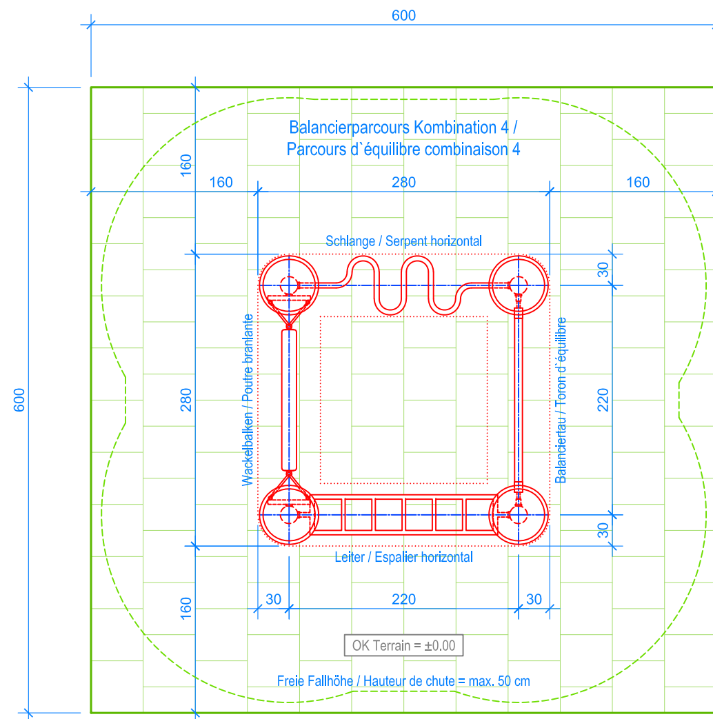
GRUNDRISS / PLAN 1:50
