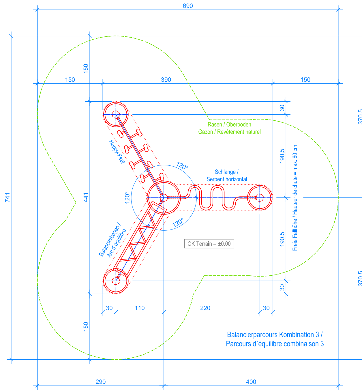
GRUNDRISS / PLAN 1:50
