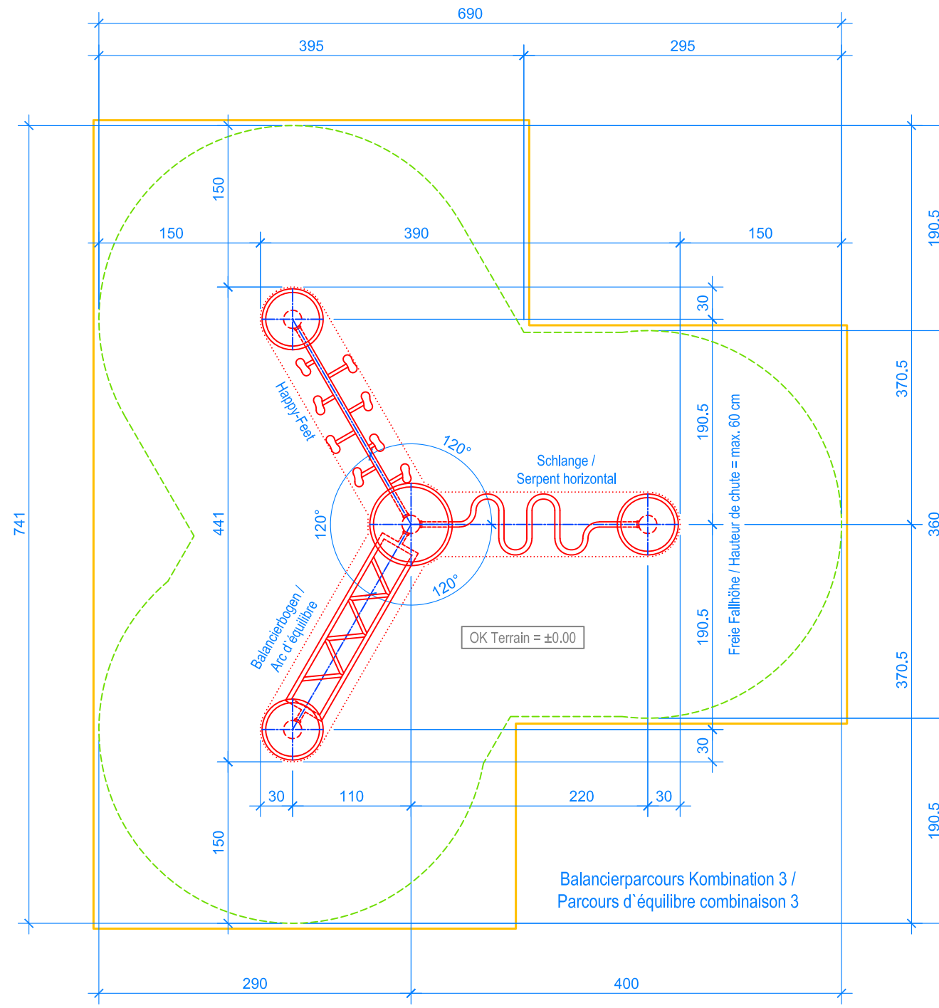
GRUNDRISS / PLAN 1:50
