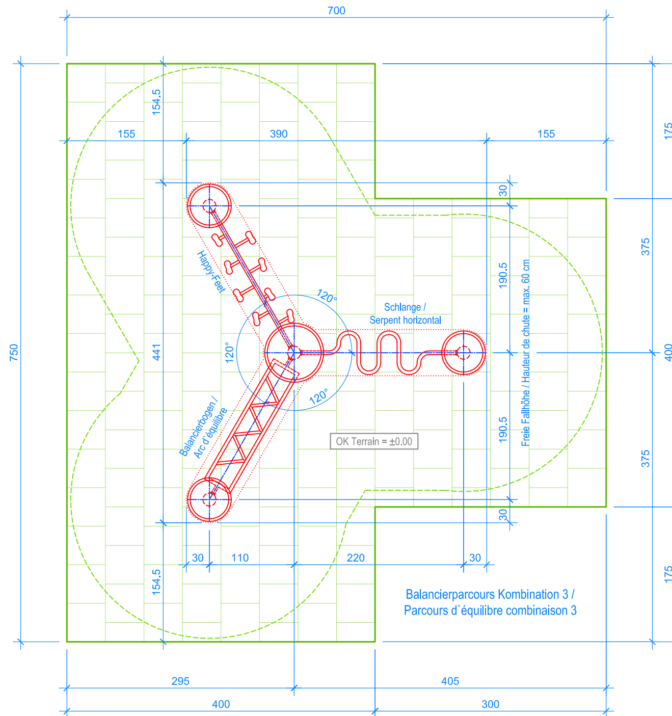
GRUNDRISS / PLAN 1:50
